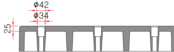
단면 A-A
